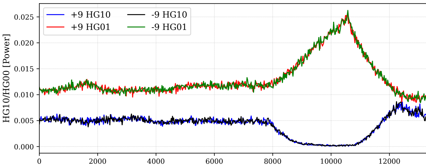
9MHz sideband mode content vs CO2
