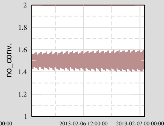
Ch 14: H0:PEM-LAB_DST2_MODE
