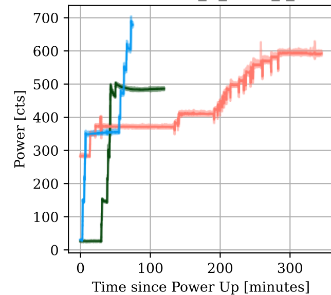
H1:LSC-POPAIR_B_RF90_I_MON
