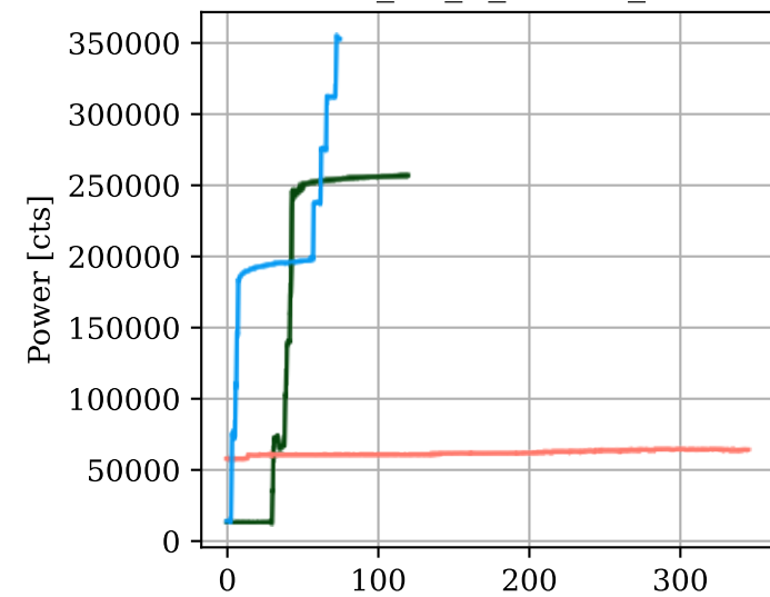
H1:LSC-POPAIR_B_RF18_I_MON
