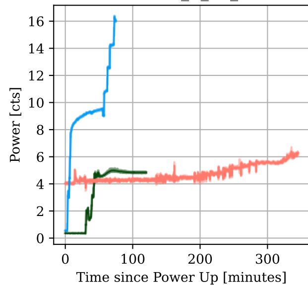
H1:LSC-REFL_B_LF_OUT16
