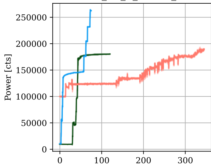
H1:LSC-REFL_A_LF_OUT16
