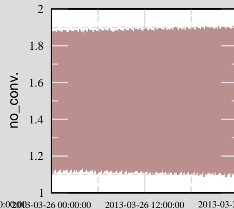
Ch 14: H0:PEM-LAB_DST2_MODE
