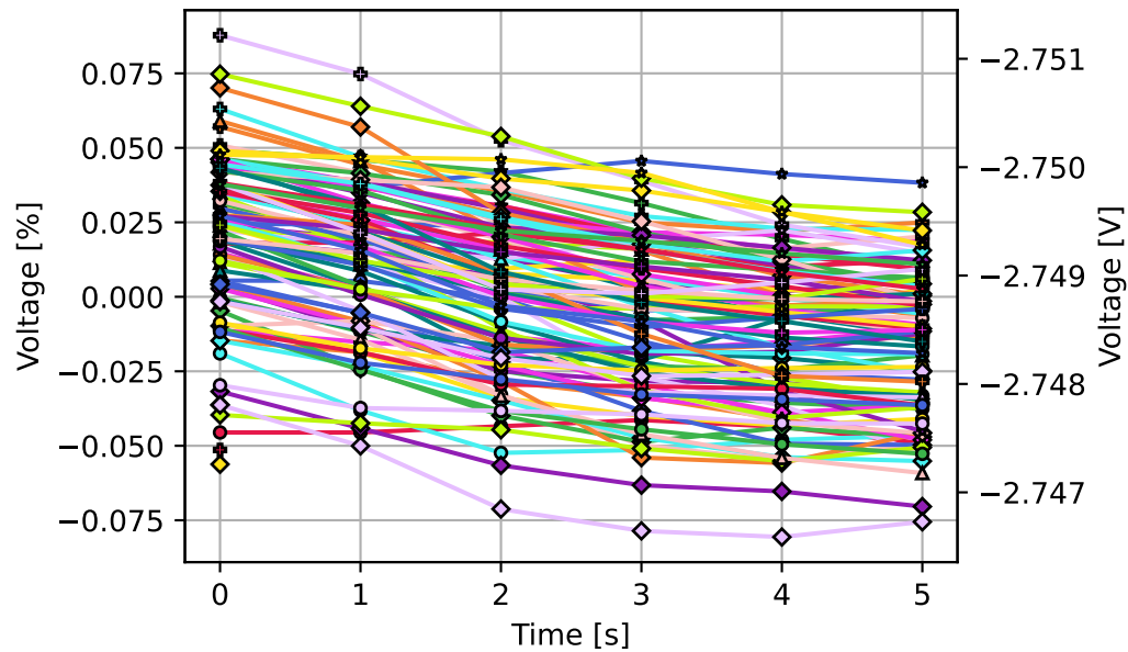
100 WSS Tran timeseries (overlaid)
