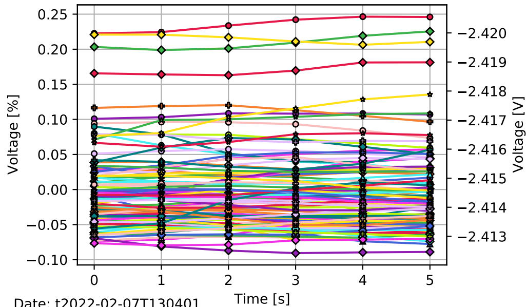
100 WSS Refl timeseries (overlaid)
