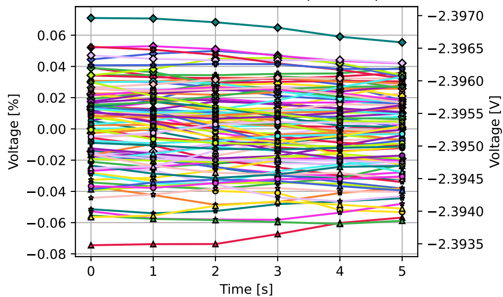
96 WSS Tran timeseries (overlaid)
