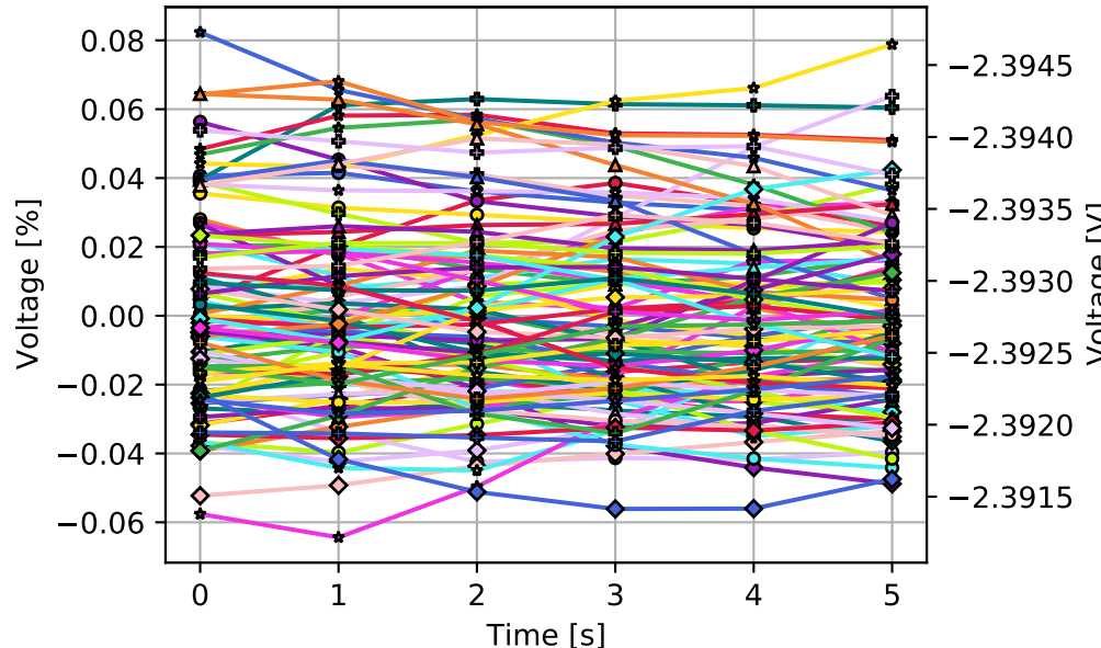
100 WSS Tran timeseries (overlaid)
