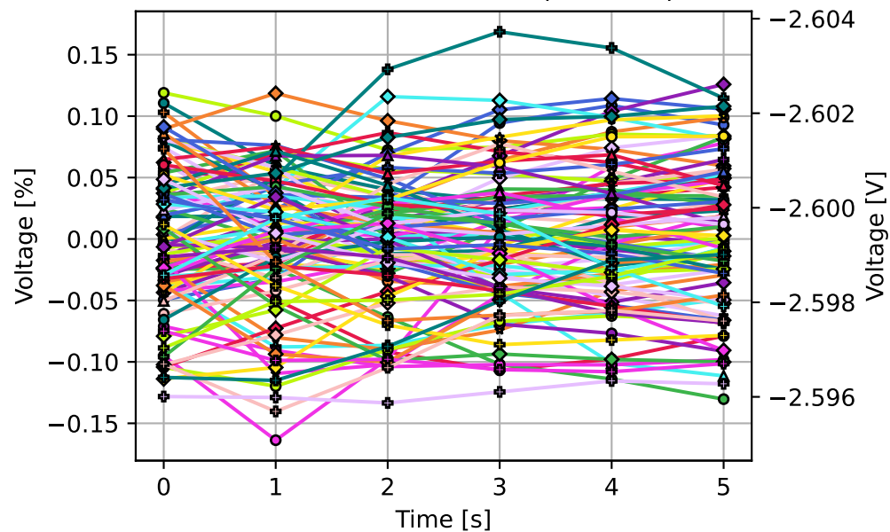
96 WSS Tran timeseries (overlaid)
