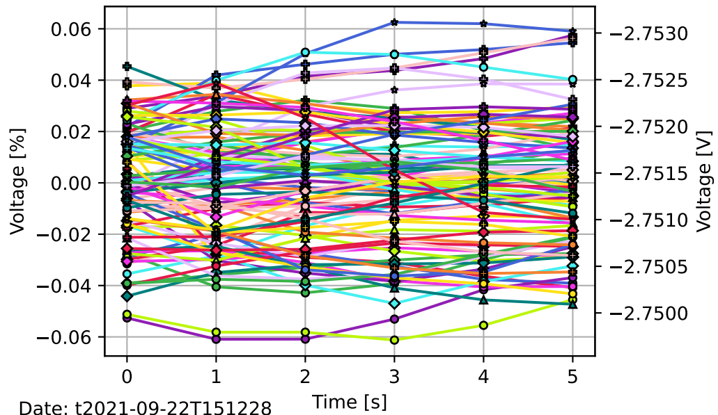
100 WSS Refl timeseries (overlaid)
