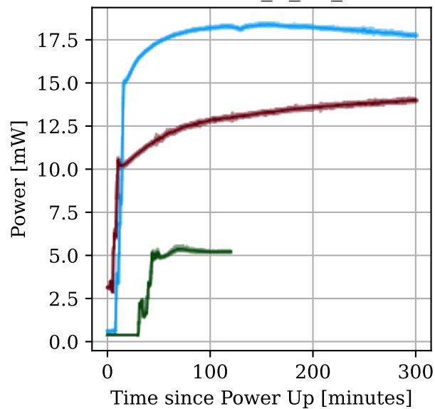
H1:LSC-REFL_A_LF_OUT16
