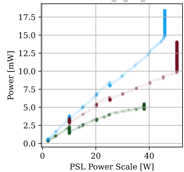
H1:LSC-REFL_A_LF_OUT16
