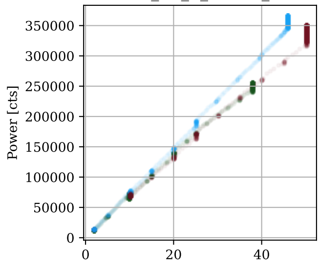
H1:LSC-POPAIR_B_RF18_I_MON
