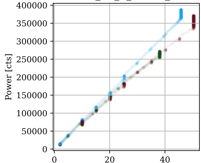
H1:LSC-POPAIR_B_RF90_I_MON
