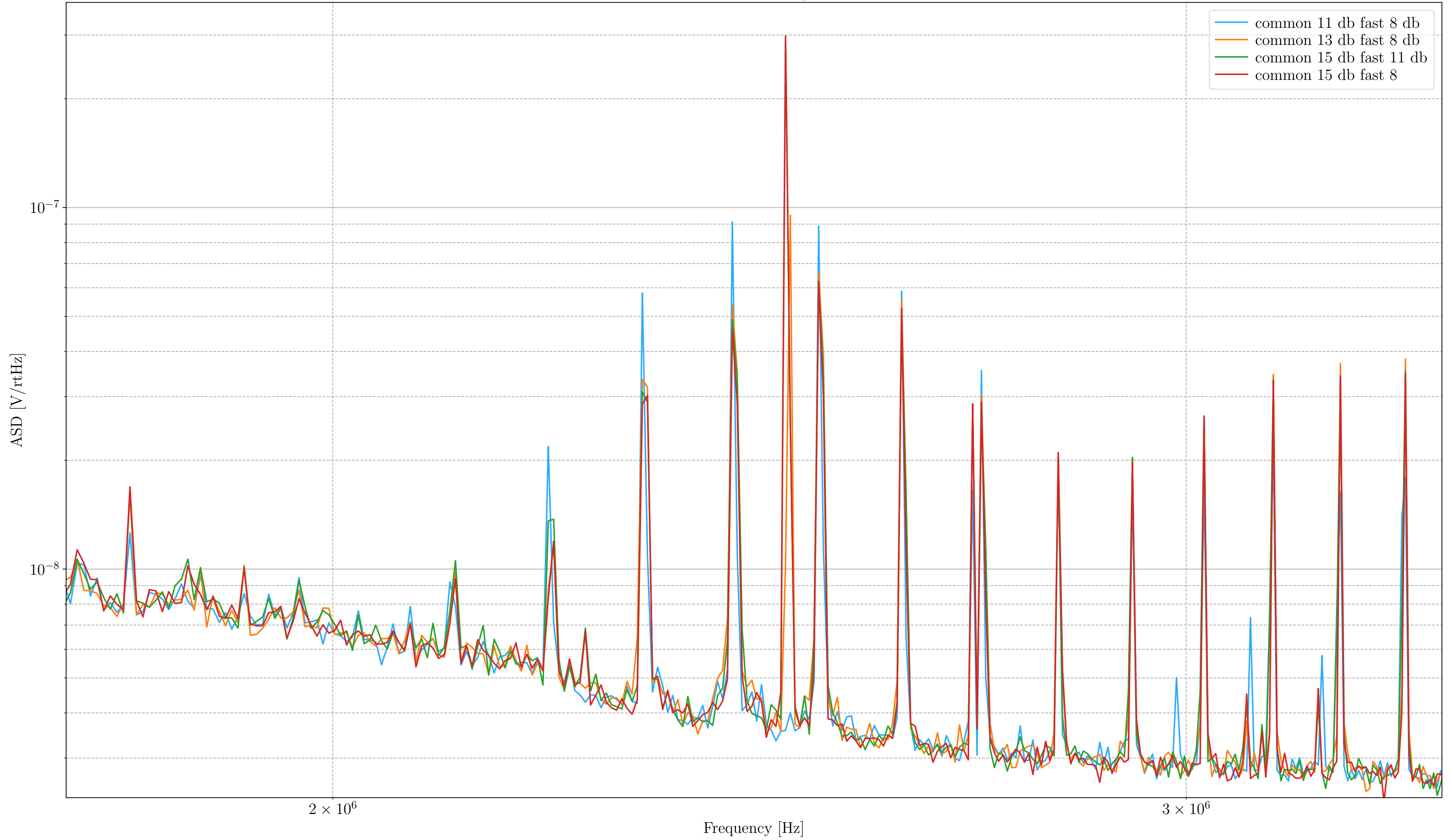
TTFSS IN1 error spectra
