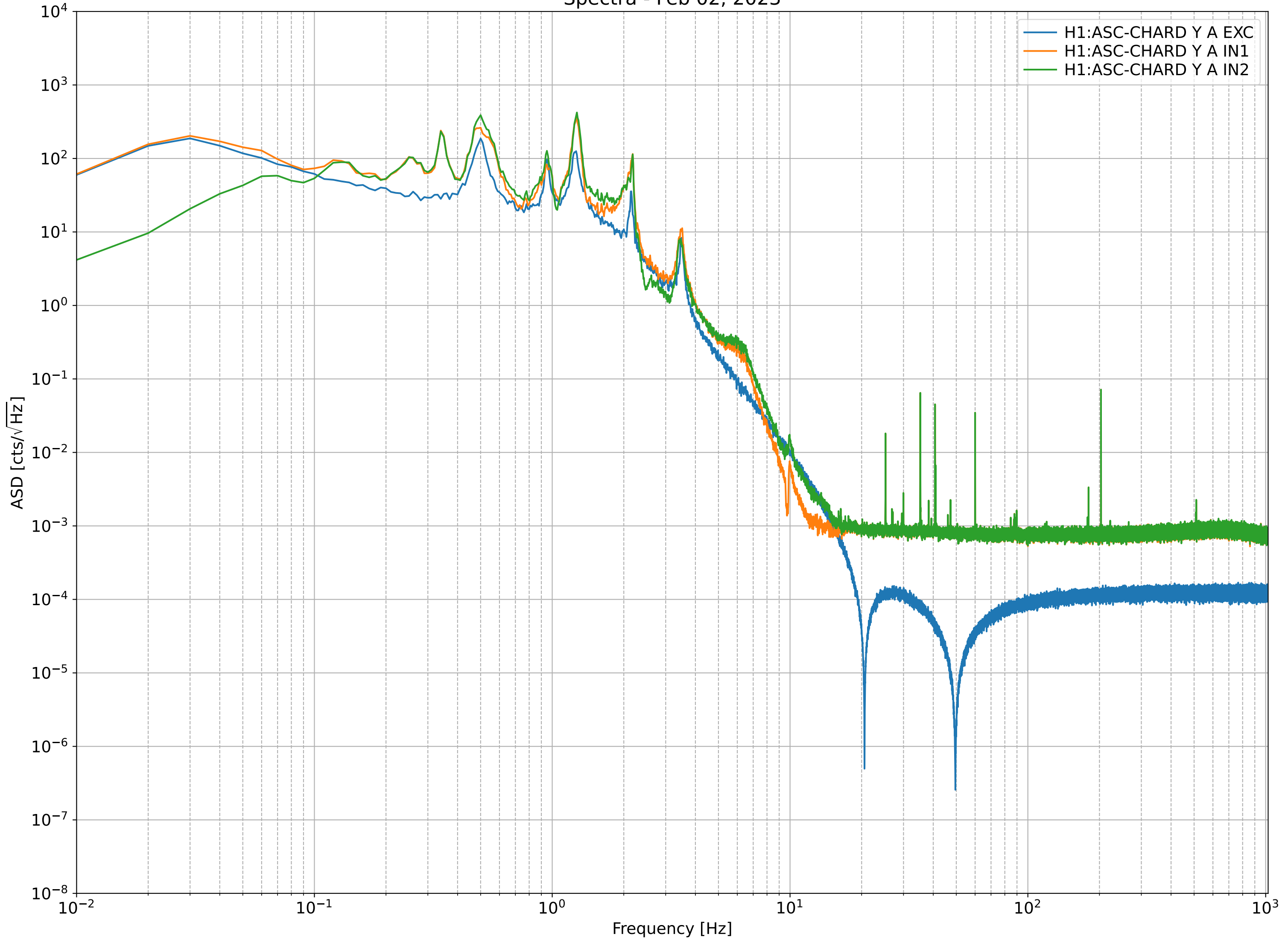
Spectra -Feb 02, 2023
