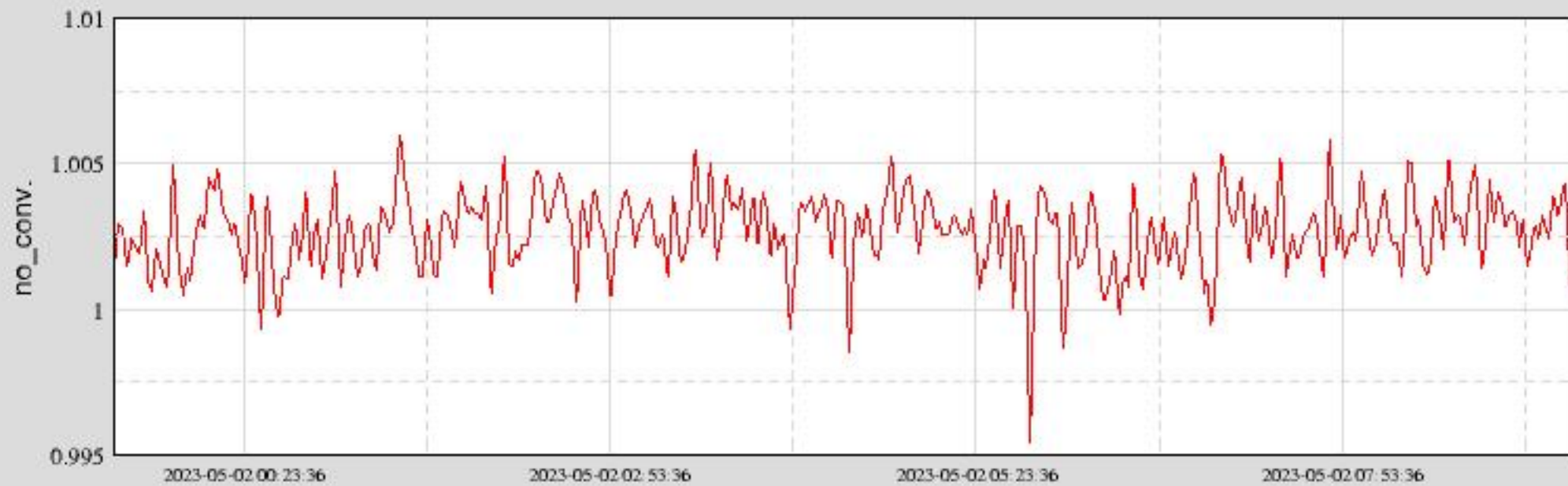
Ch 1: H1:CAL-CS_TDEP_PCAL_X_OVER_Y_REL_MAG
