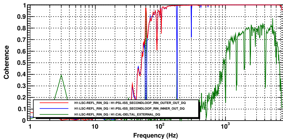
Coherence
