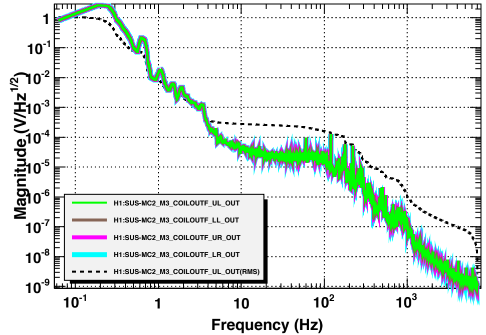
Amplitude Spectral Density - DAC Output Signal, H1 SUS MC2
