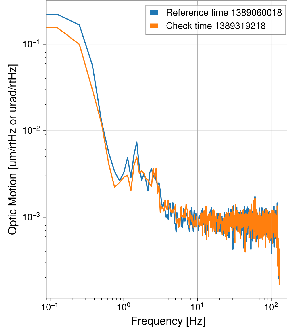
H1:SUS-BS_M1_DAMP_P_IN1_DQ
