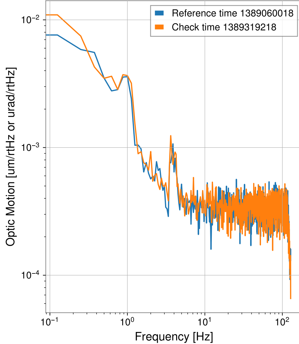
H1:SUS-MC3_M1_DAMP_Y_IN1_DQ
