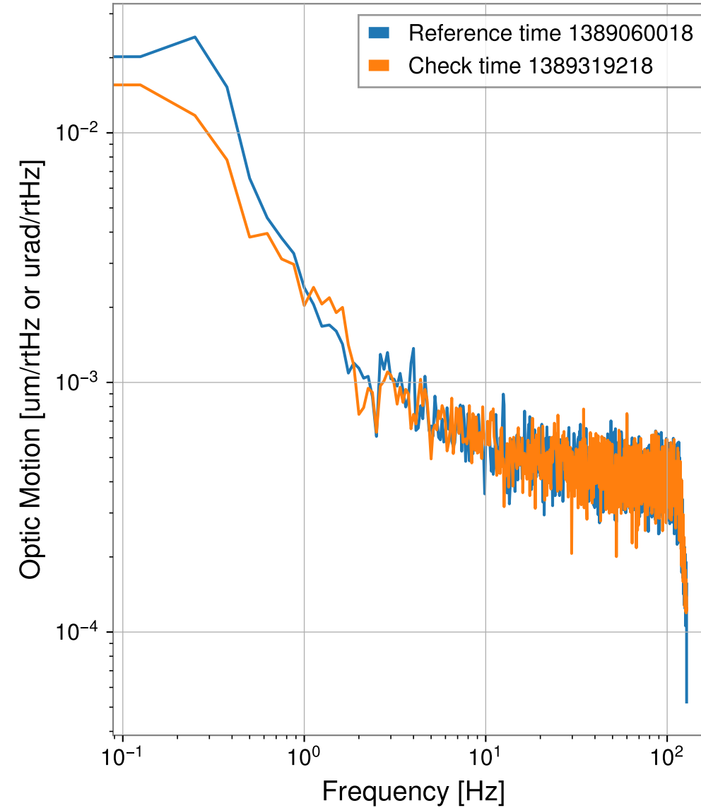
H1:SUS-SR3_M1_DAMP_R_IN1_DQ
