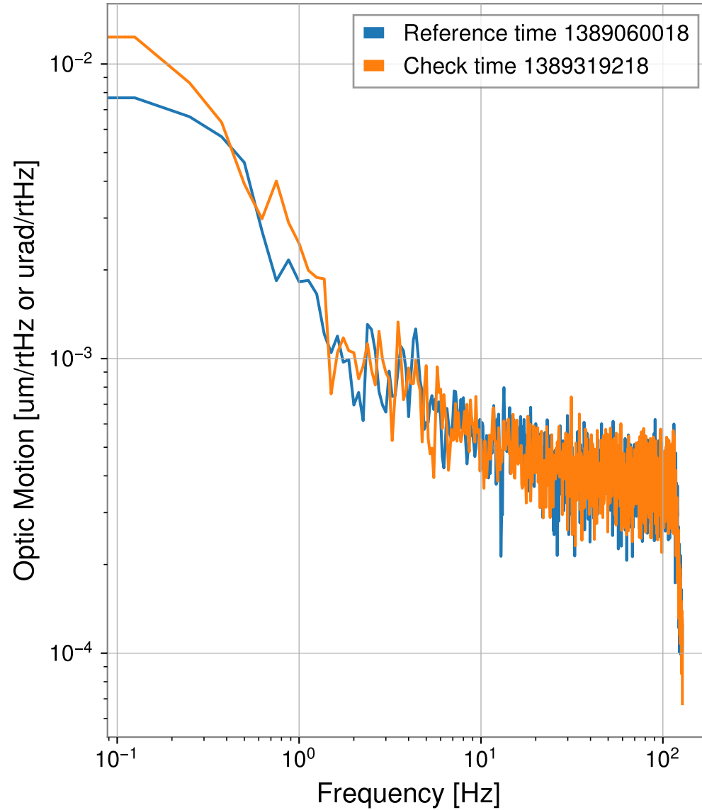
H1:SUS-SR3_M1_DAMP_Y_IN1_DQ
