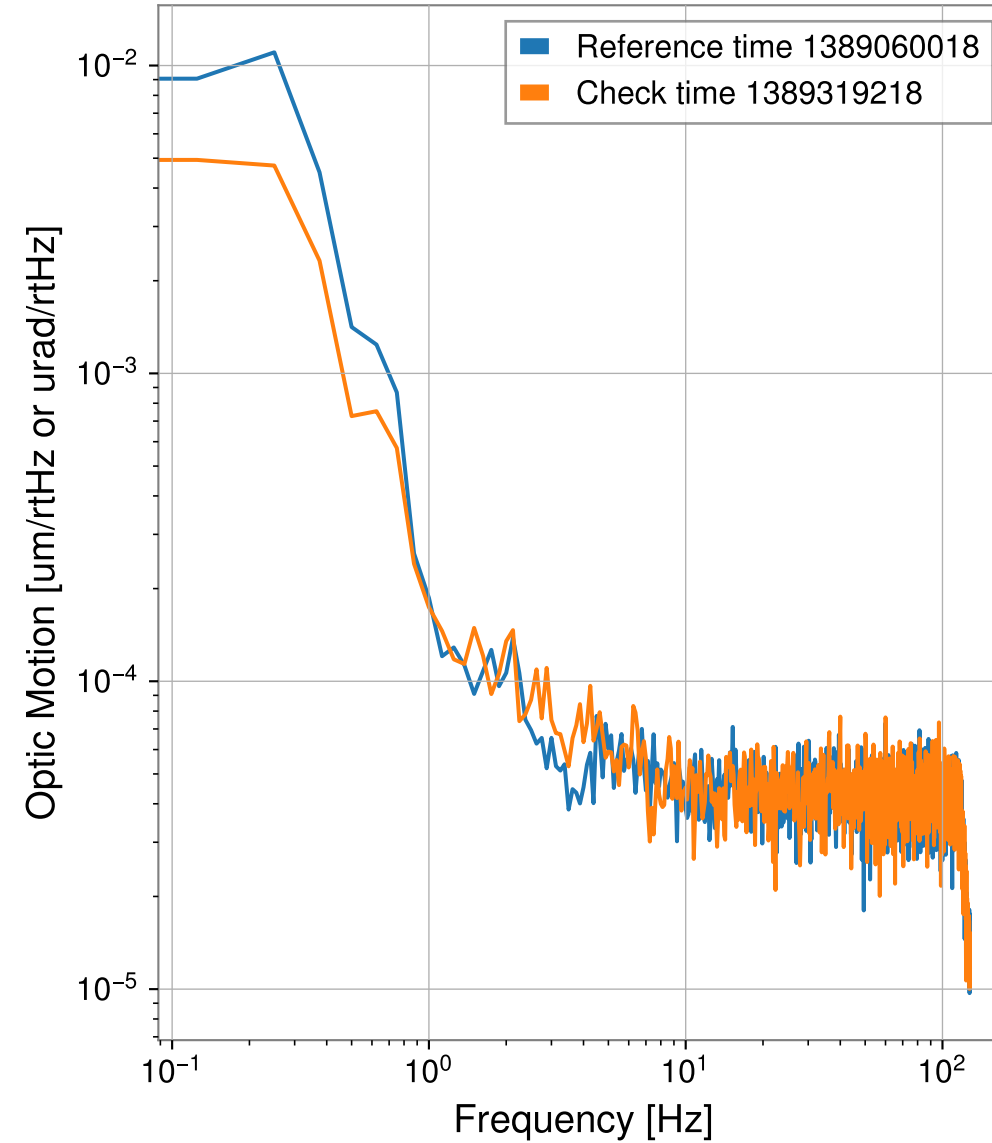
H1:SUS-SR3_M1_DAMP_T_IN1_DQ
