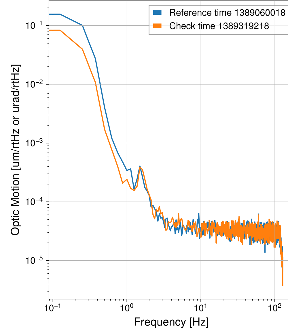
H1:SUS-BS_M1_DAMP_L_IN1_DQ
