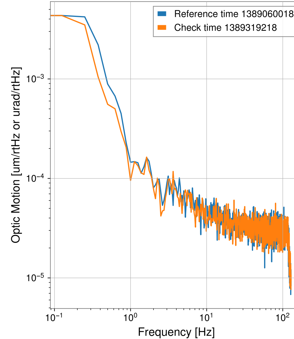
H1:SUS-SR3_M1_DAMP_L_IN1_DQ
