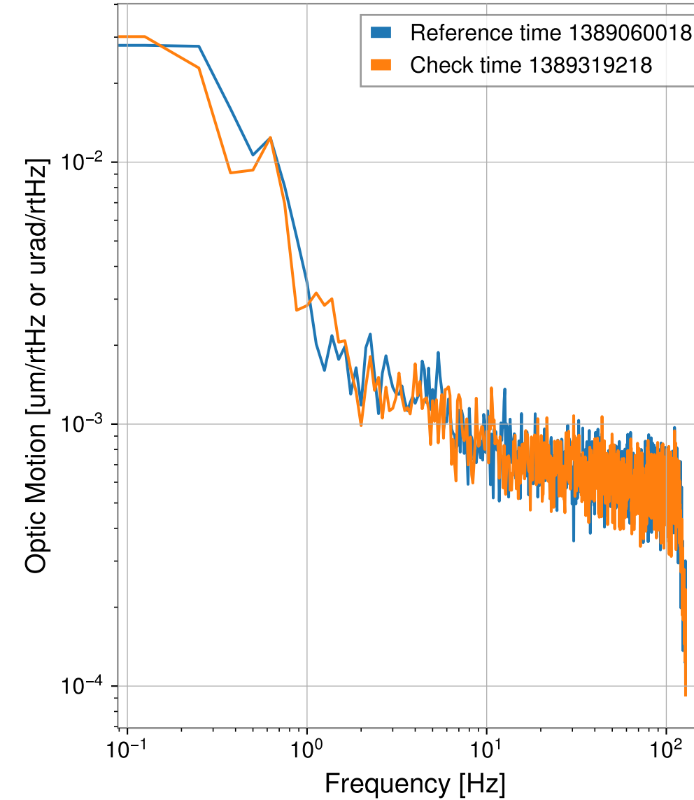
H1:SUS-SR3_M1_DAMP_P_IN1_DQ
