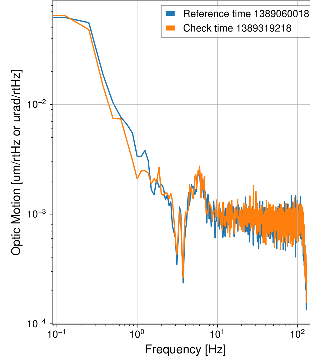
H1:SUS-MC3_M1_DAMP_P_IN1_DQ
