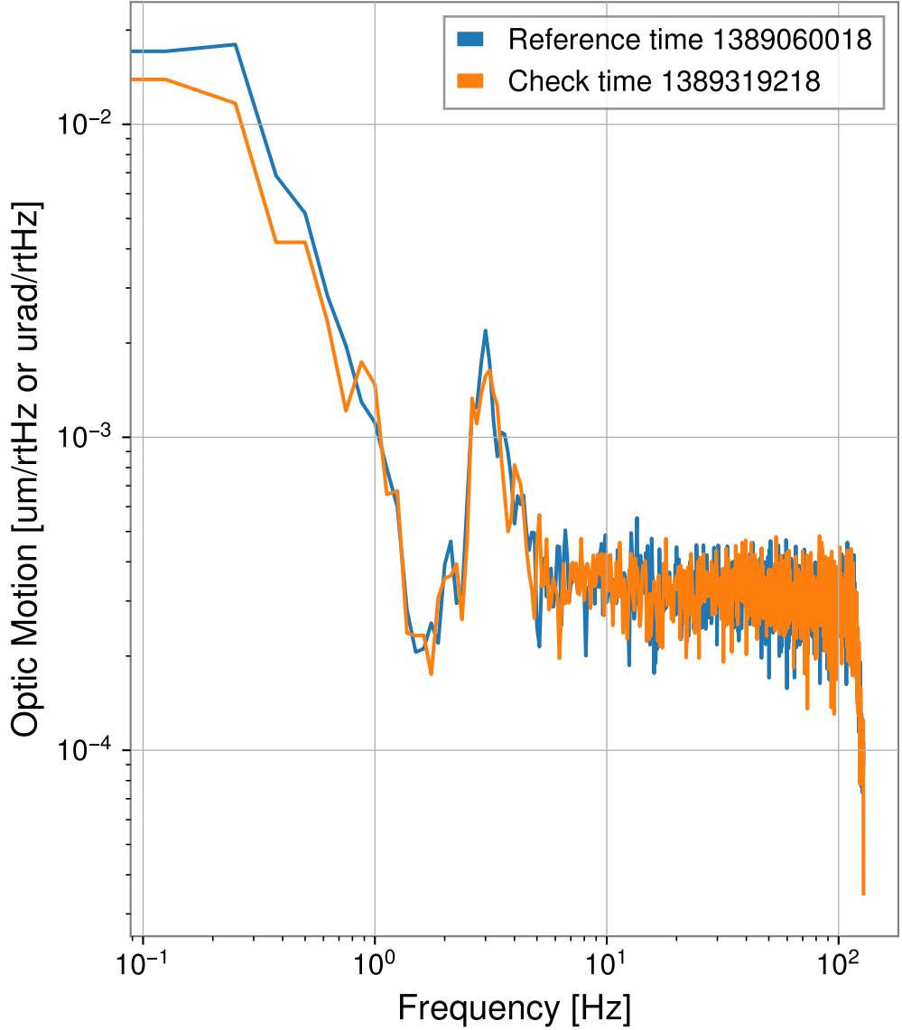
H1:SUS-BS_M1_DAMP_Y_IN1_DQ
