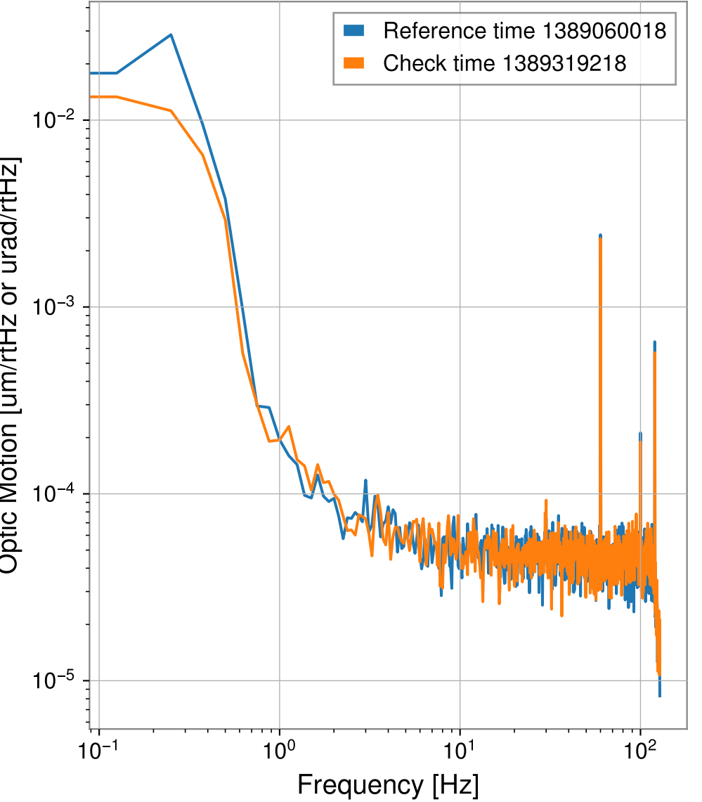
H1:SUS-BS_M1_DAMP_T_IN1_DQ
