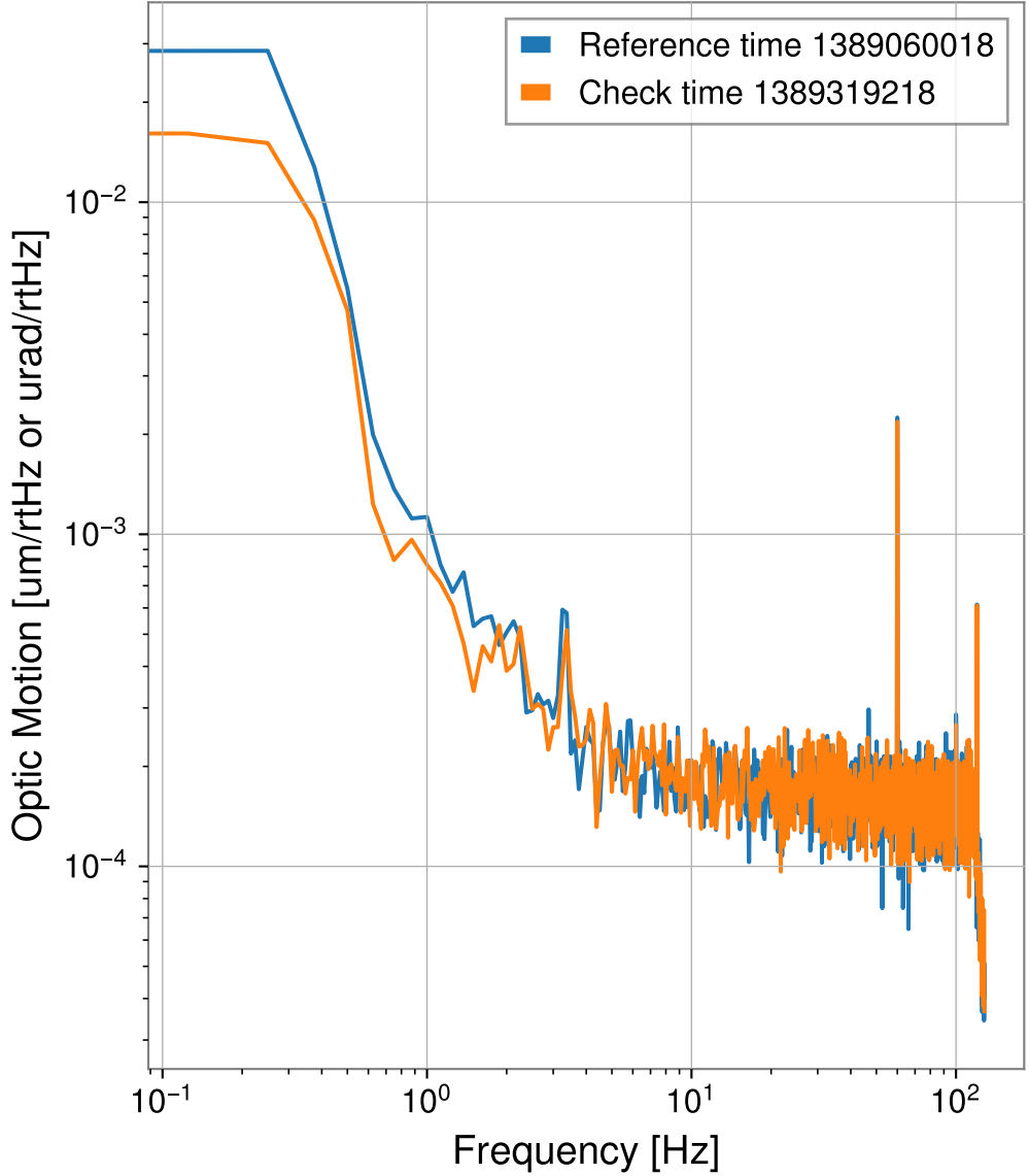
H1:SUS-BS_M1_DAMP_R_IN1_DQ
