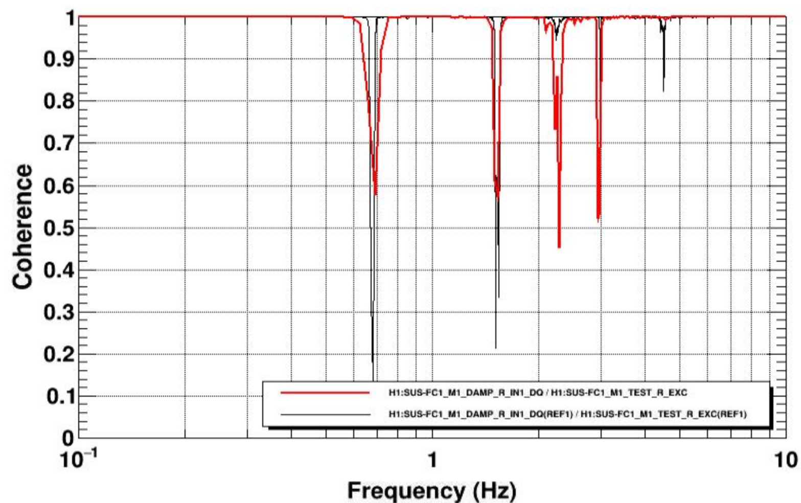
Coherence
