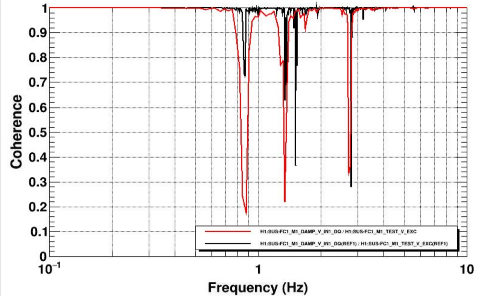
Coherence
