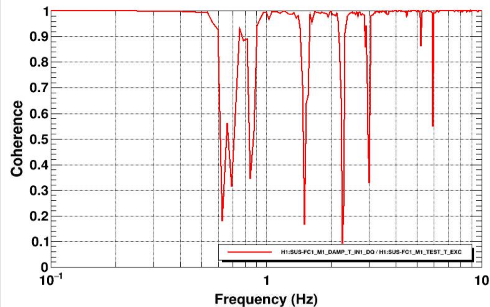
Coherence
