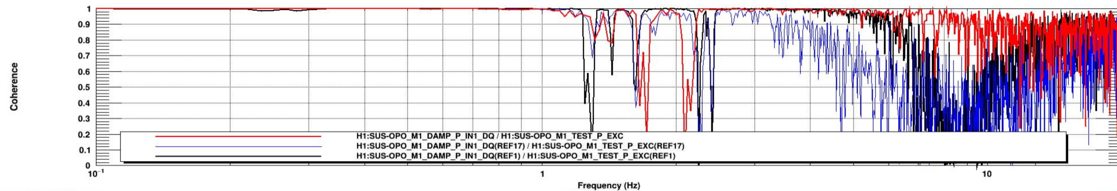
Coherence
