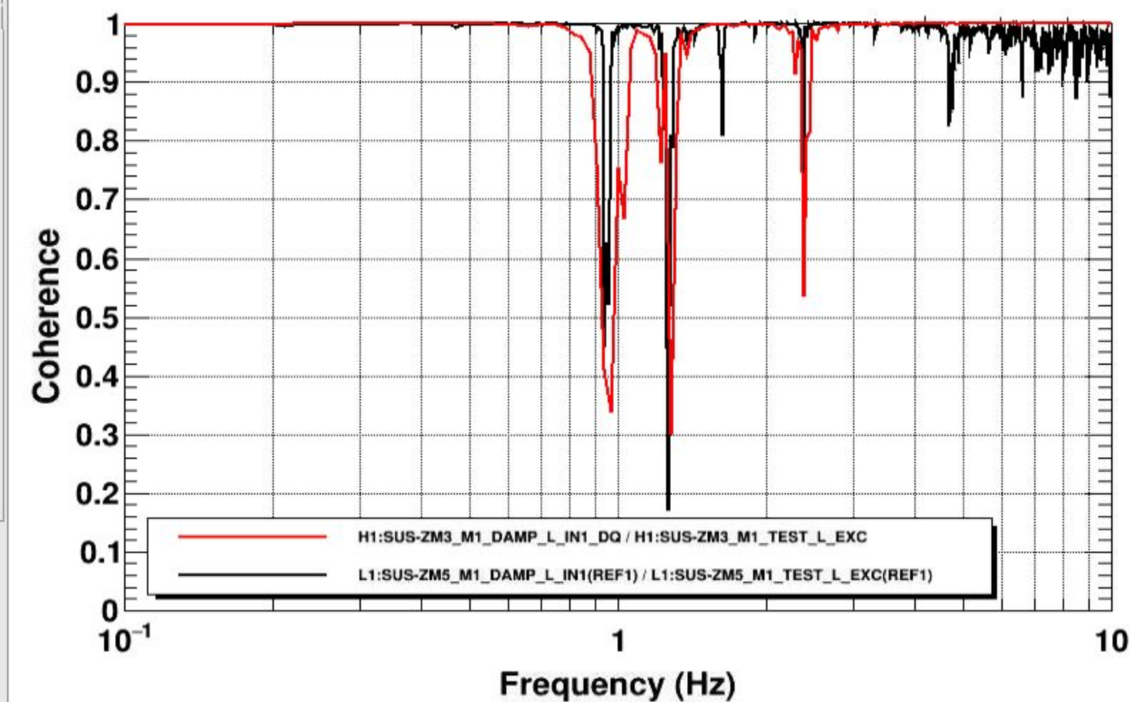
Coherence
