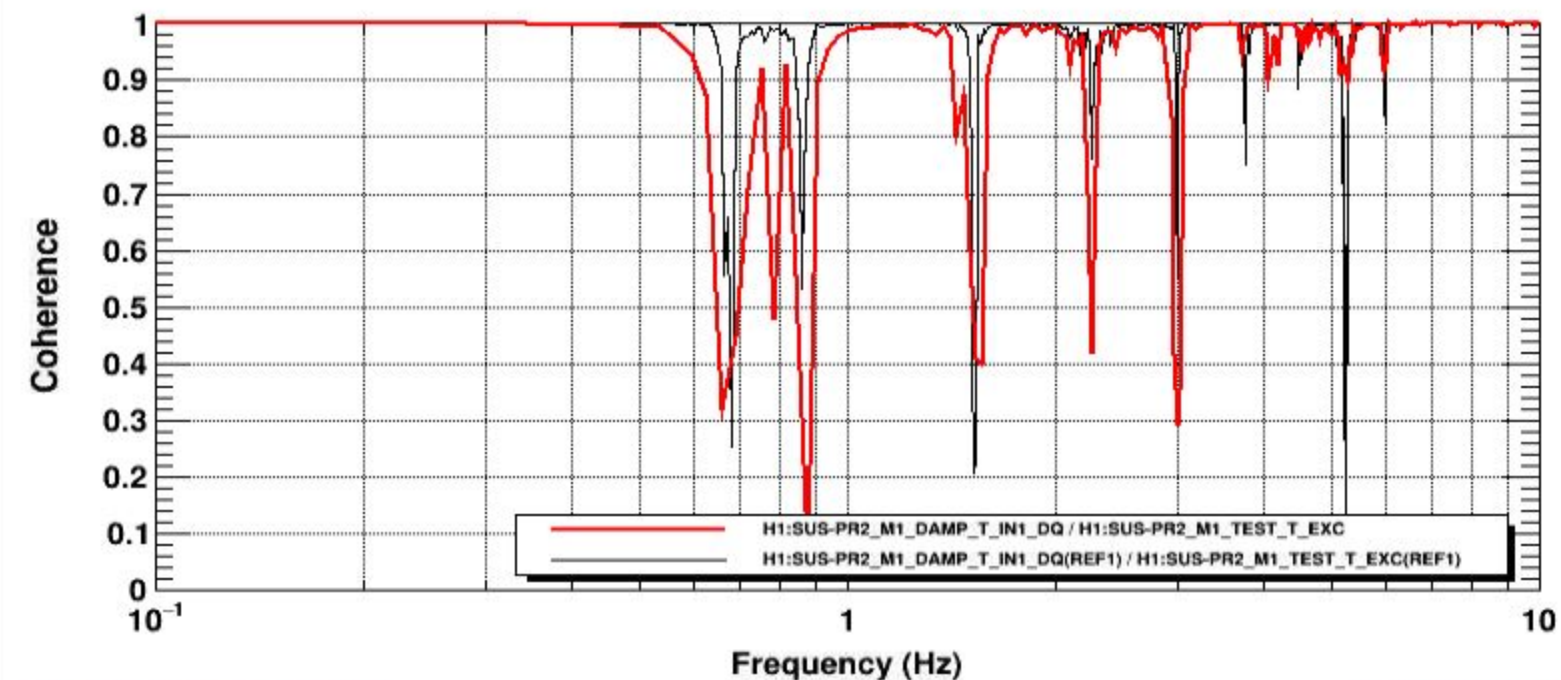
Coherence
