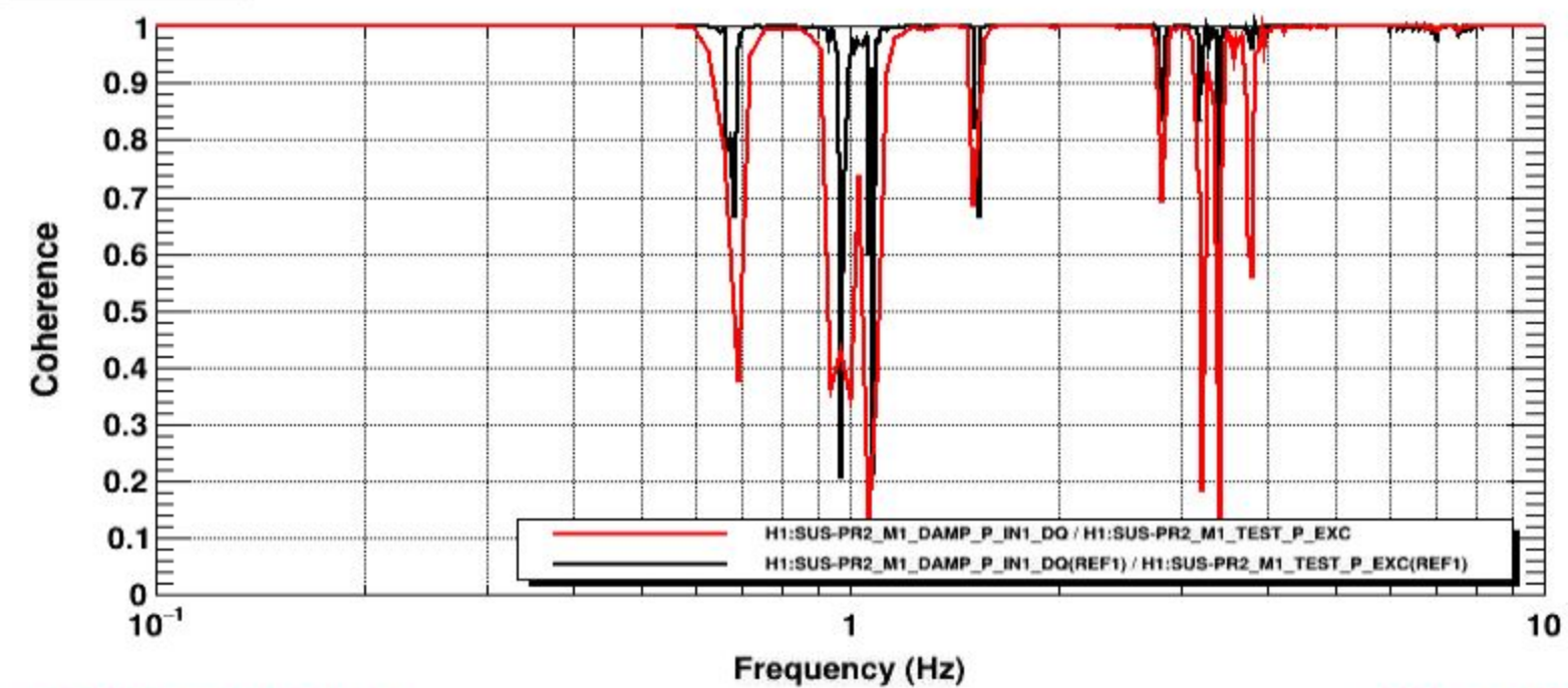
Coherence
