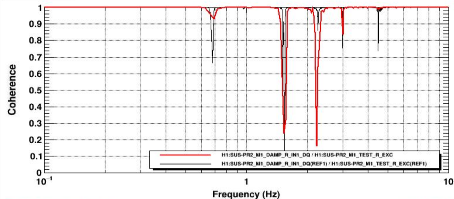
Coherence
