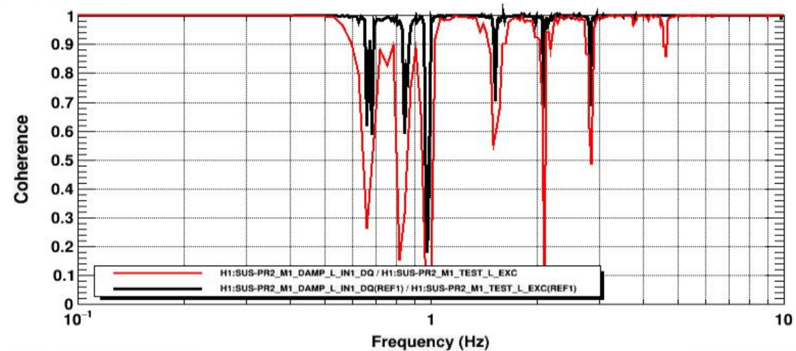
Coherence
