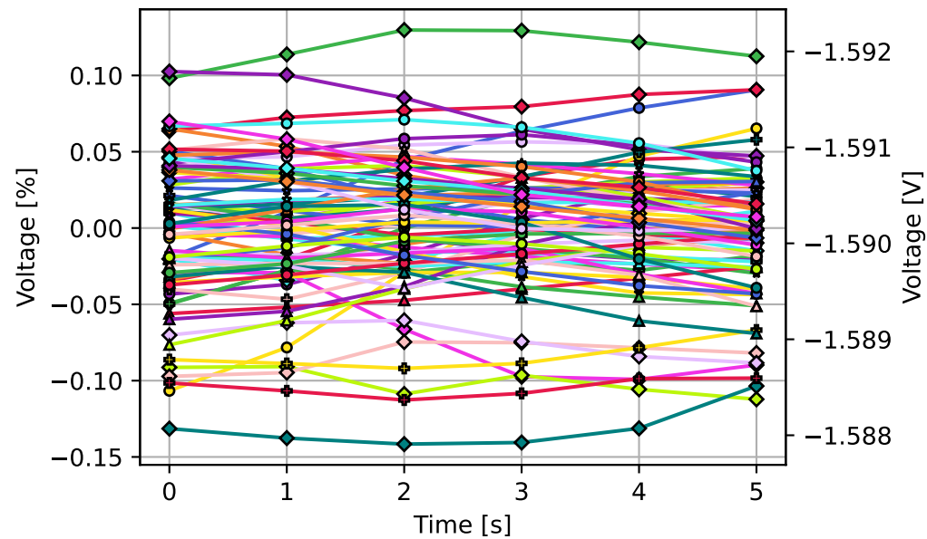
80 PS5 Tran timeseries (overlaid)
