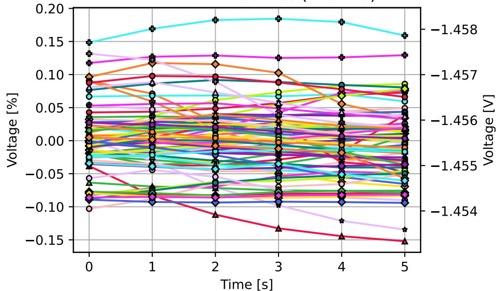
80 PS5 Refl timeseries (overlaid)
