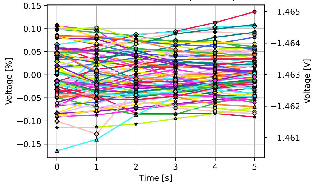
80 PS5 Tran timeseries (overlaid)
