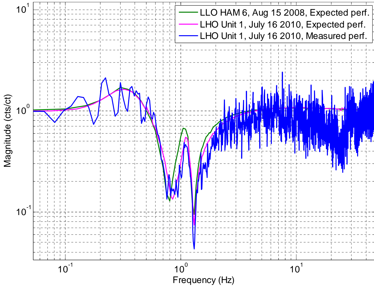
HAM-ISI Dampig loop sensitivity ('Undamped'/'Damped' )
