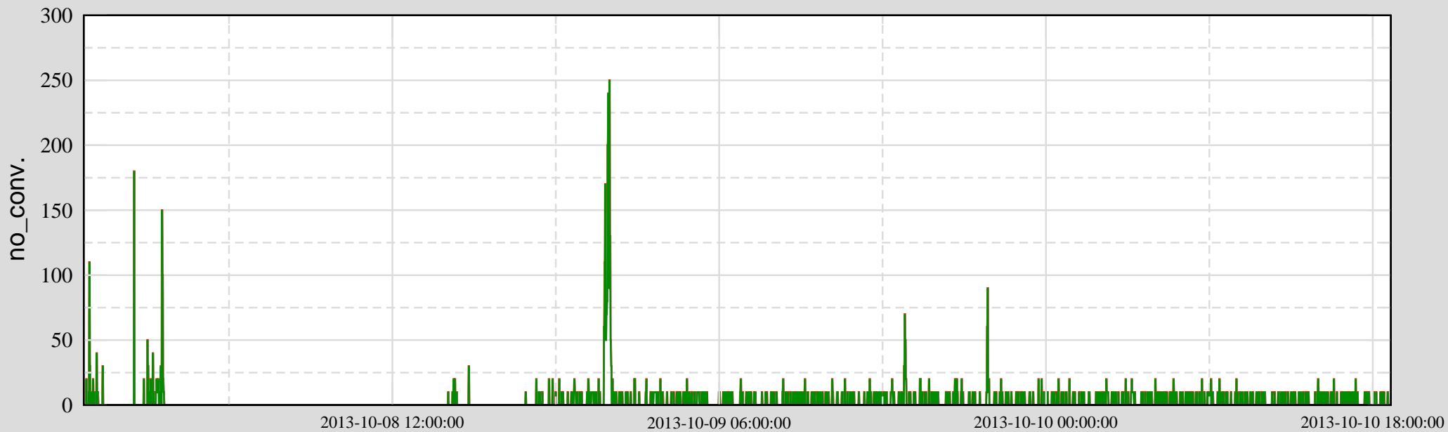
Ch 2: H0:PEM-CS_DUST_LAB2_500NM_PCF
