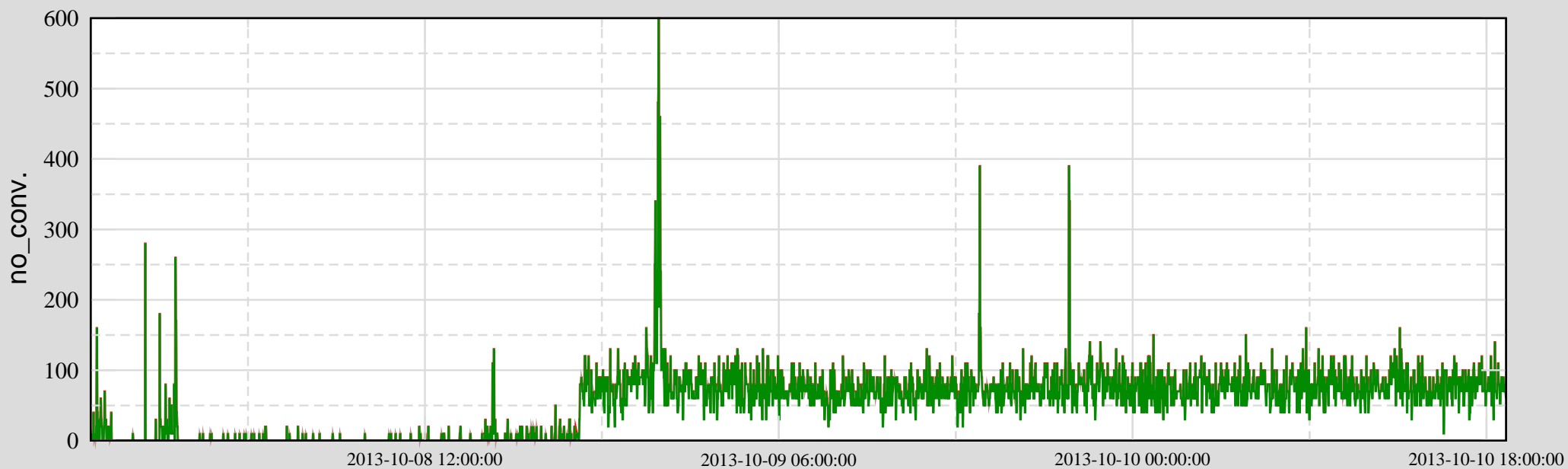
Ch 1: H0:PEM-CS_DUST_LAB2_300NM_PCF
