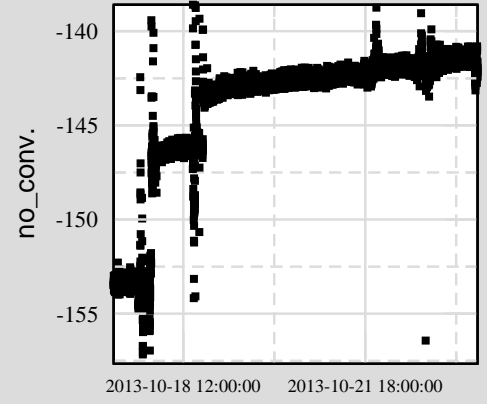
Ch 1: H1:SUS-ETMX_M0_DAMP_Y_IN1_DQ Ch 6: H1:SUS-ETMX_L1_OSEMINF_LL_OUT_DQ Ch 9: H1:SUS-ETMX_L2_OSEMINF_UL_OUT_DQ Ch 12: H1:SUS-ETMX_L2_OSEMINF_LR_OUT_DQ
