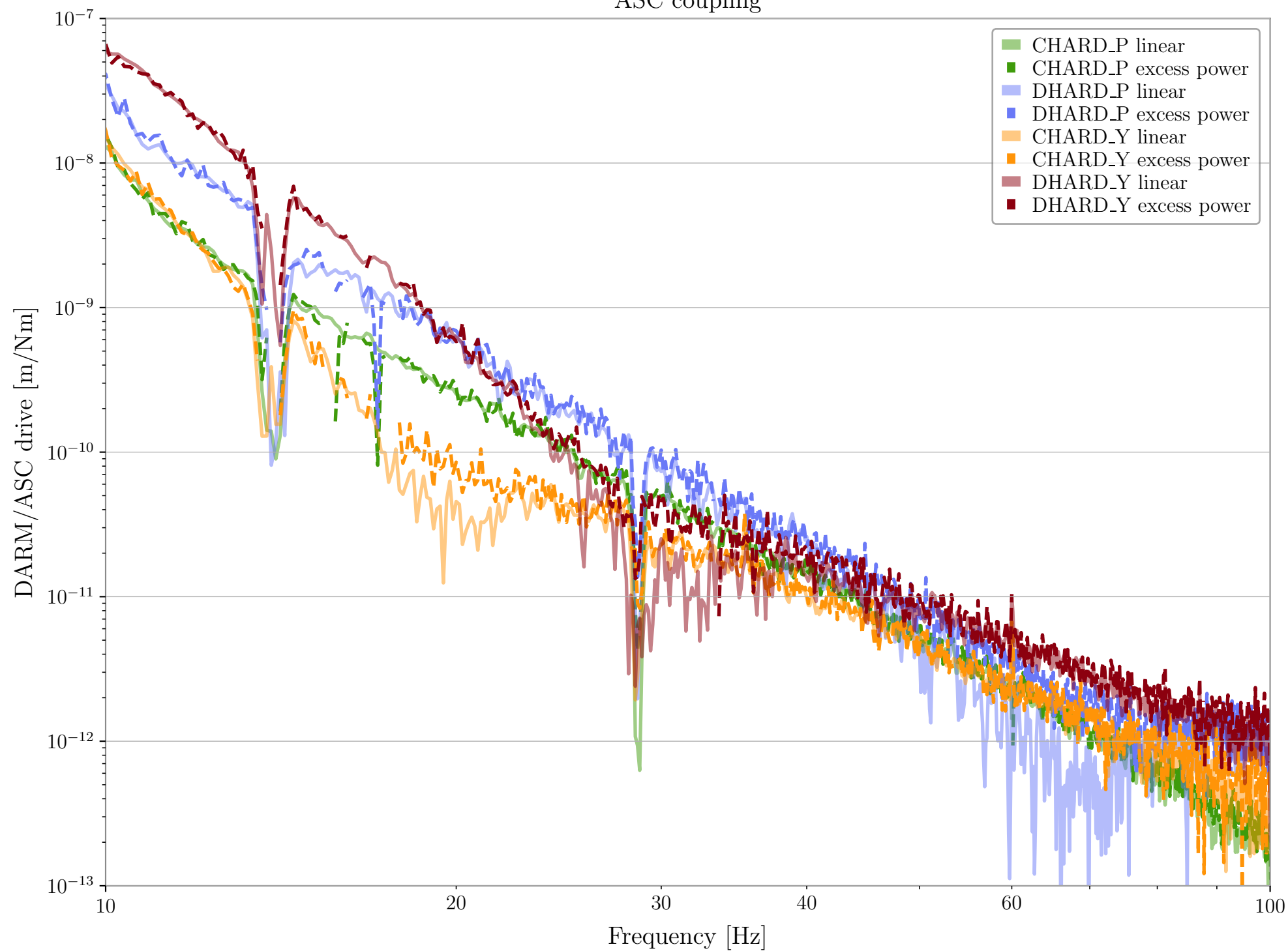
ASC coupling
