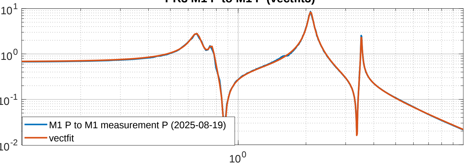
PR3 M1 P to M1 P (vectfit3)
