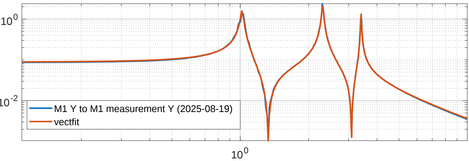
PR3 M1 Y to M1 Y (vectfit3)
