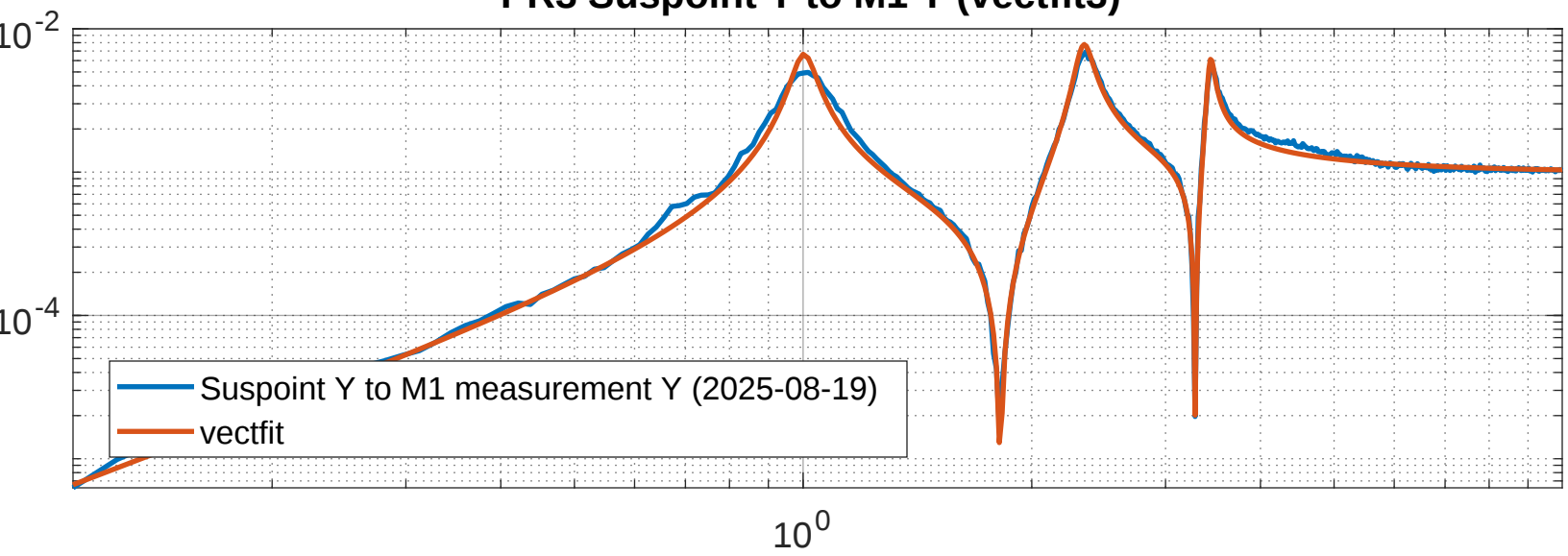
PR3 Suspoint Y to M1 Y (vectfit3)
