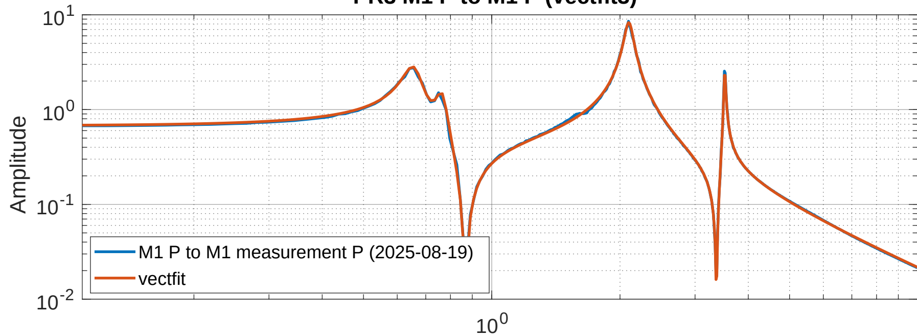
PR3 M1 P to M1 P (vectfit3)
