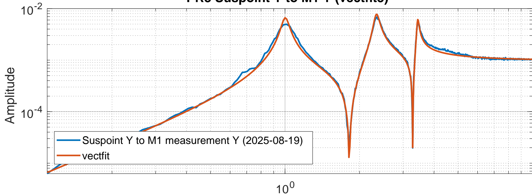
PR3 Suspoint Y to M1 Y (vectfit3)
