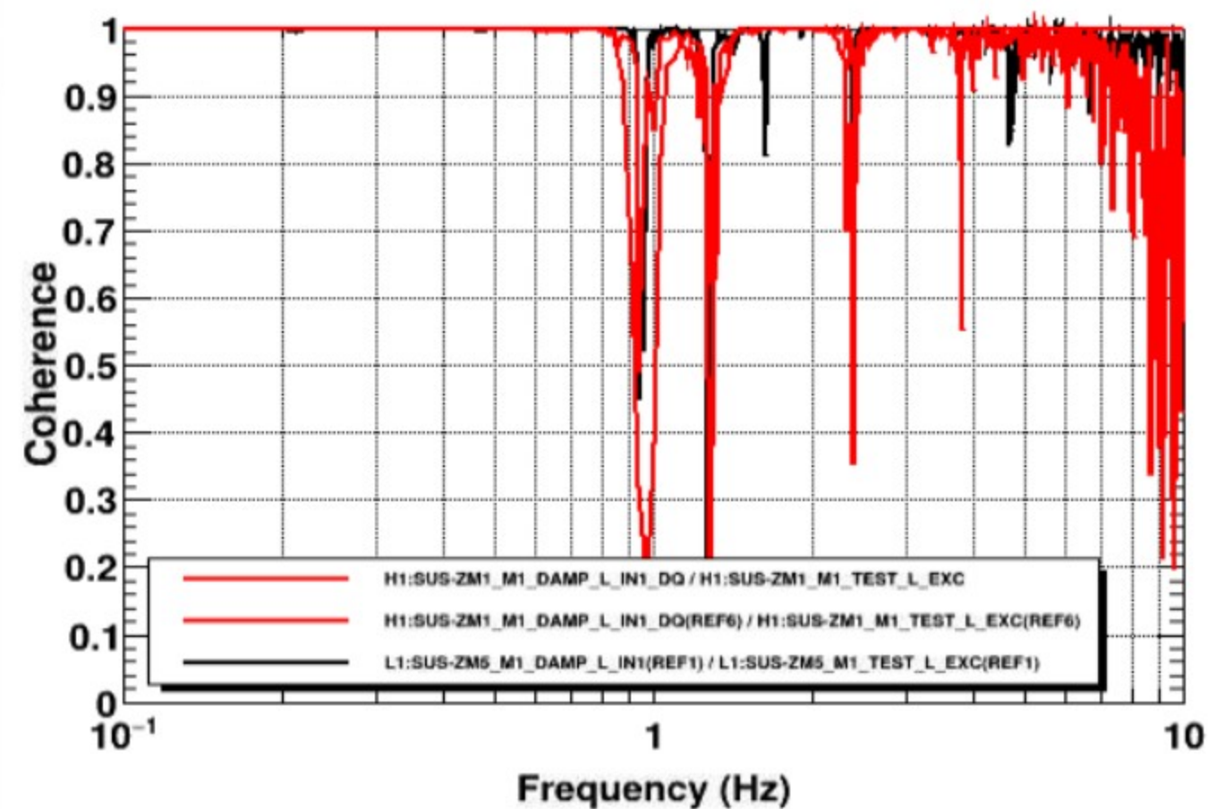
Coherence
