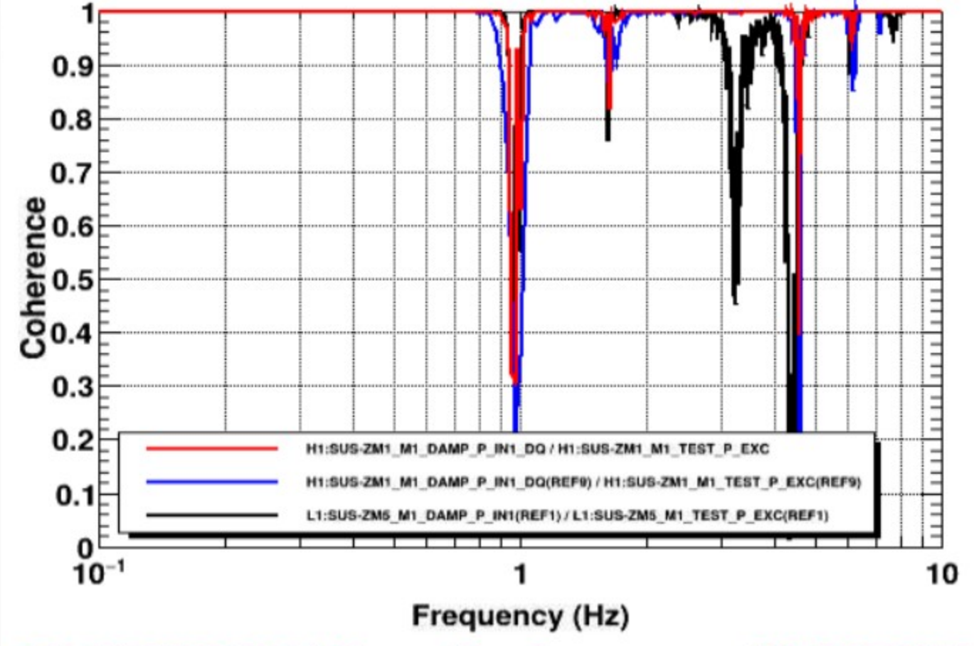
Coherence
