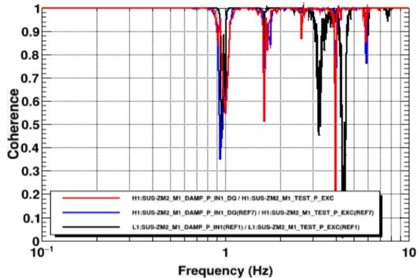
Coherence
