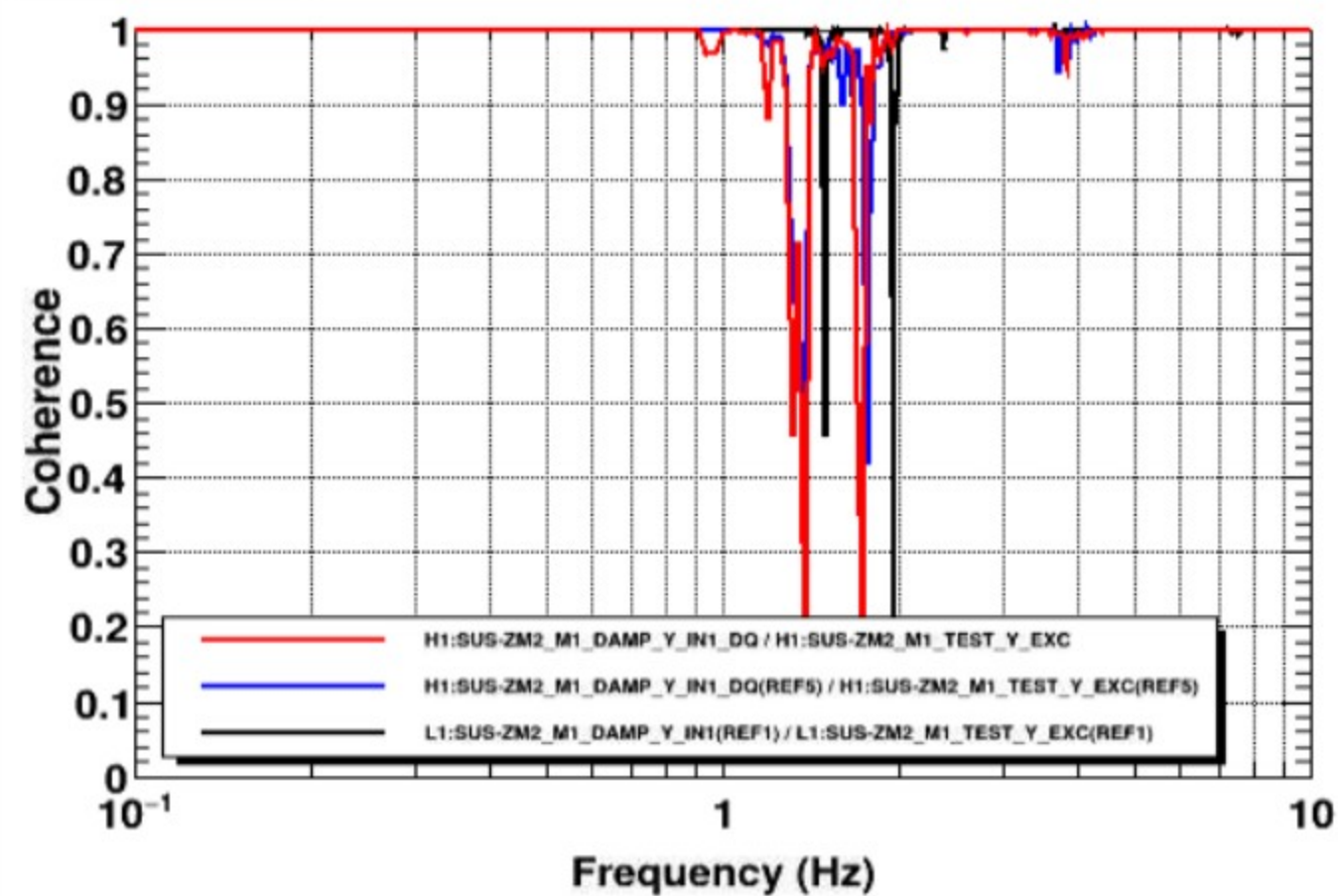
Coherence
