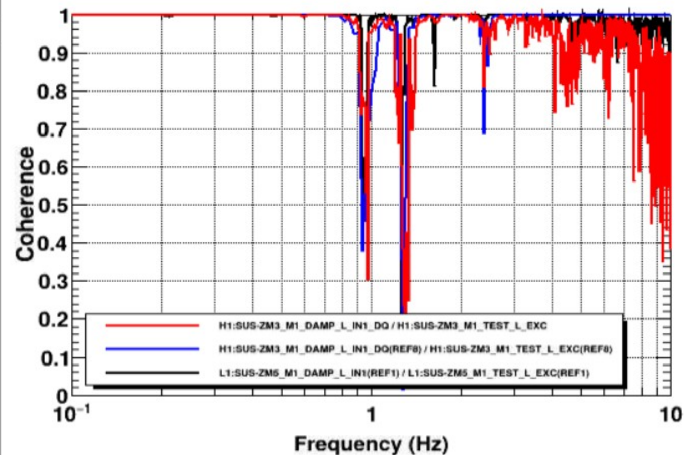
Coherence
