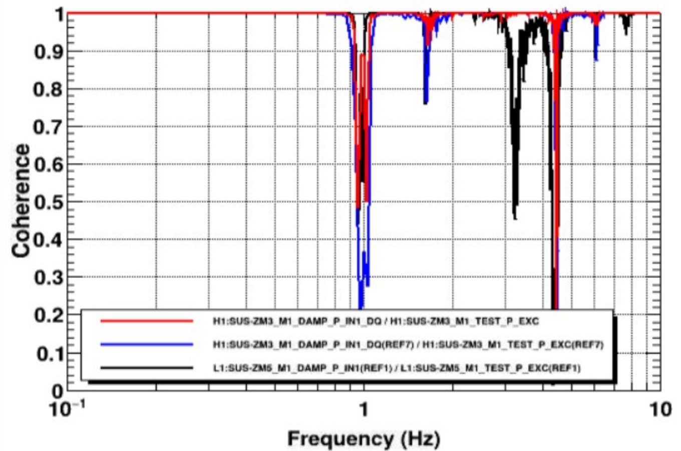
Coherence
