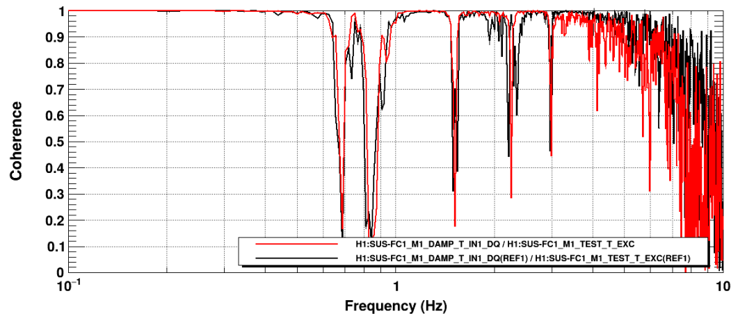
Coherence
