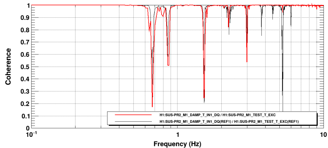
Coherence
