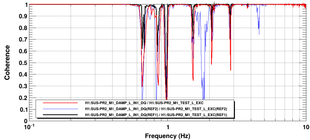
Coherence
