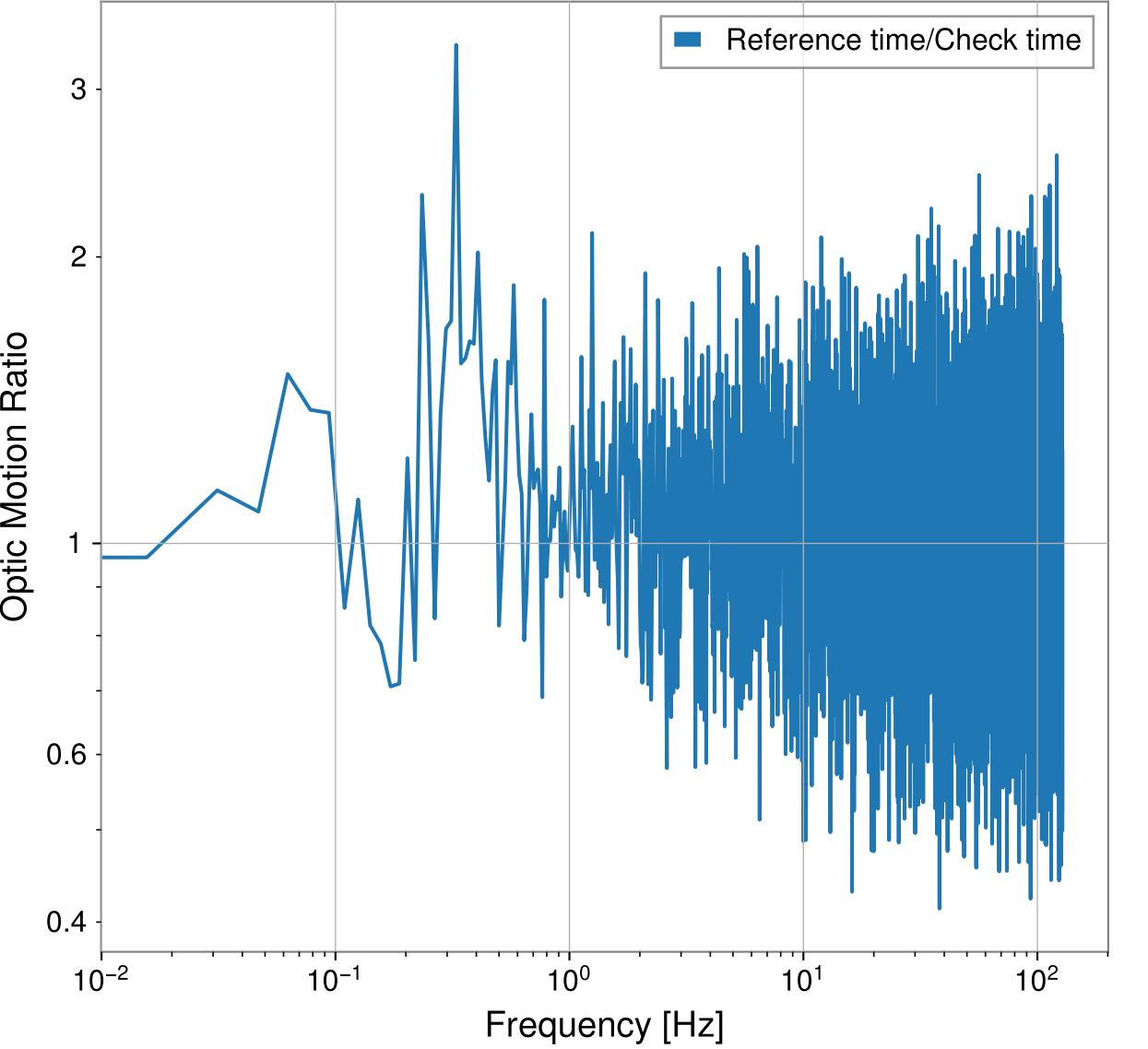
H1:SUS-TMSX_M1_DAMP_Y_IN1_DQ
