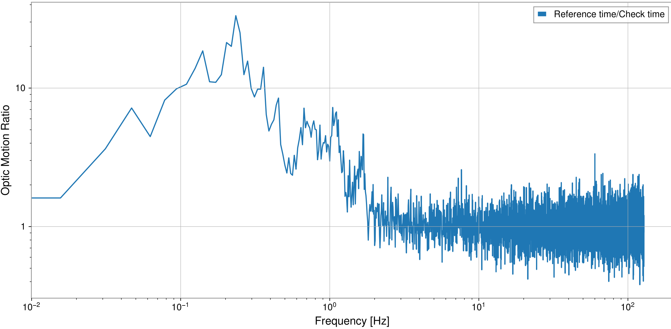
H1:SUS-RM1_M1_DAMP_Y_IN1_DQ
