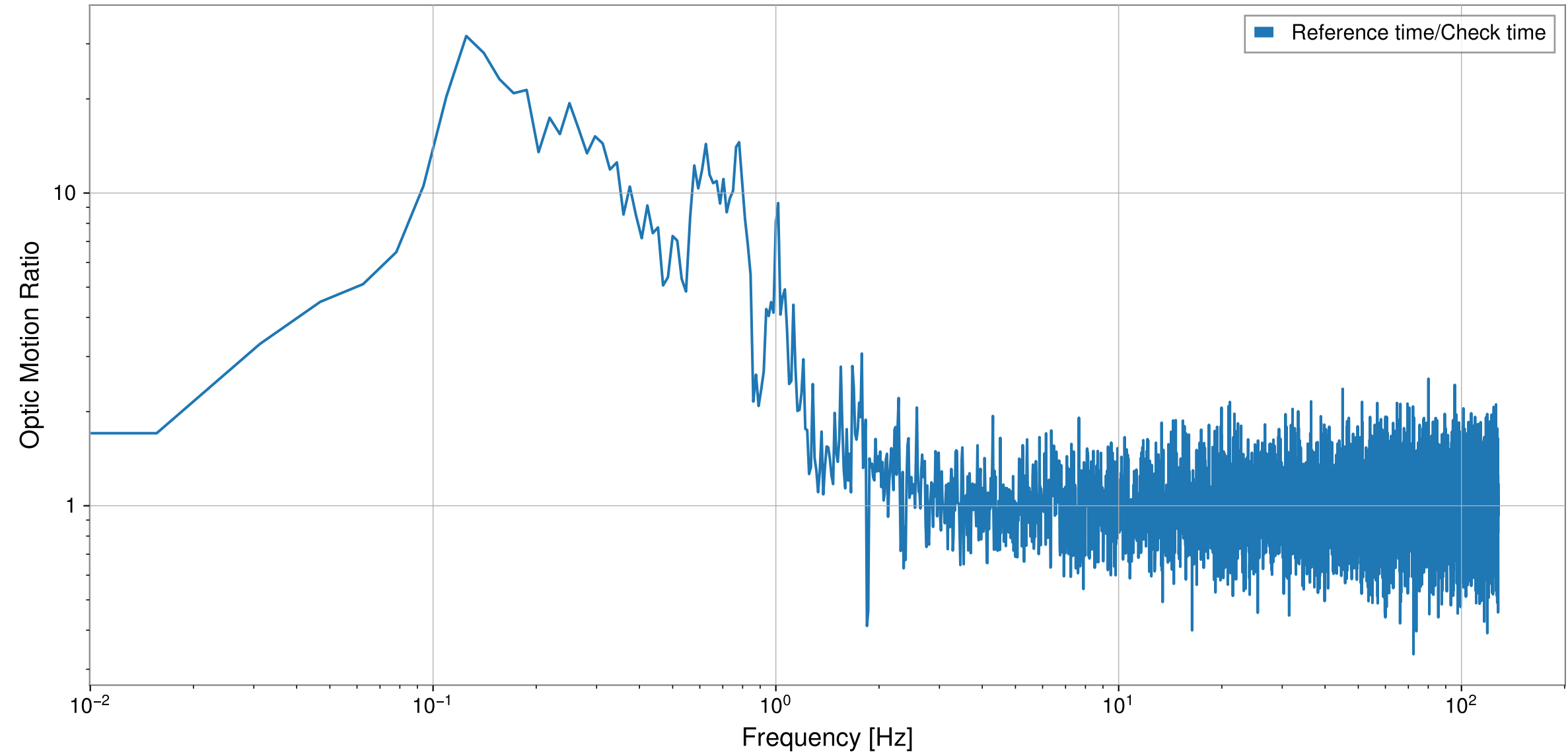
H1:SUS-RM1_M1_DAMP_P_IN1_DQ
