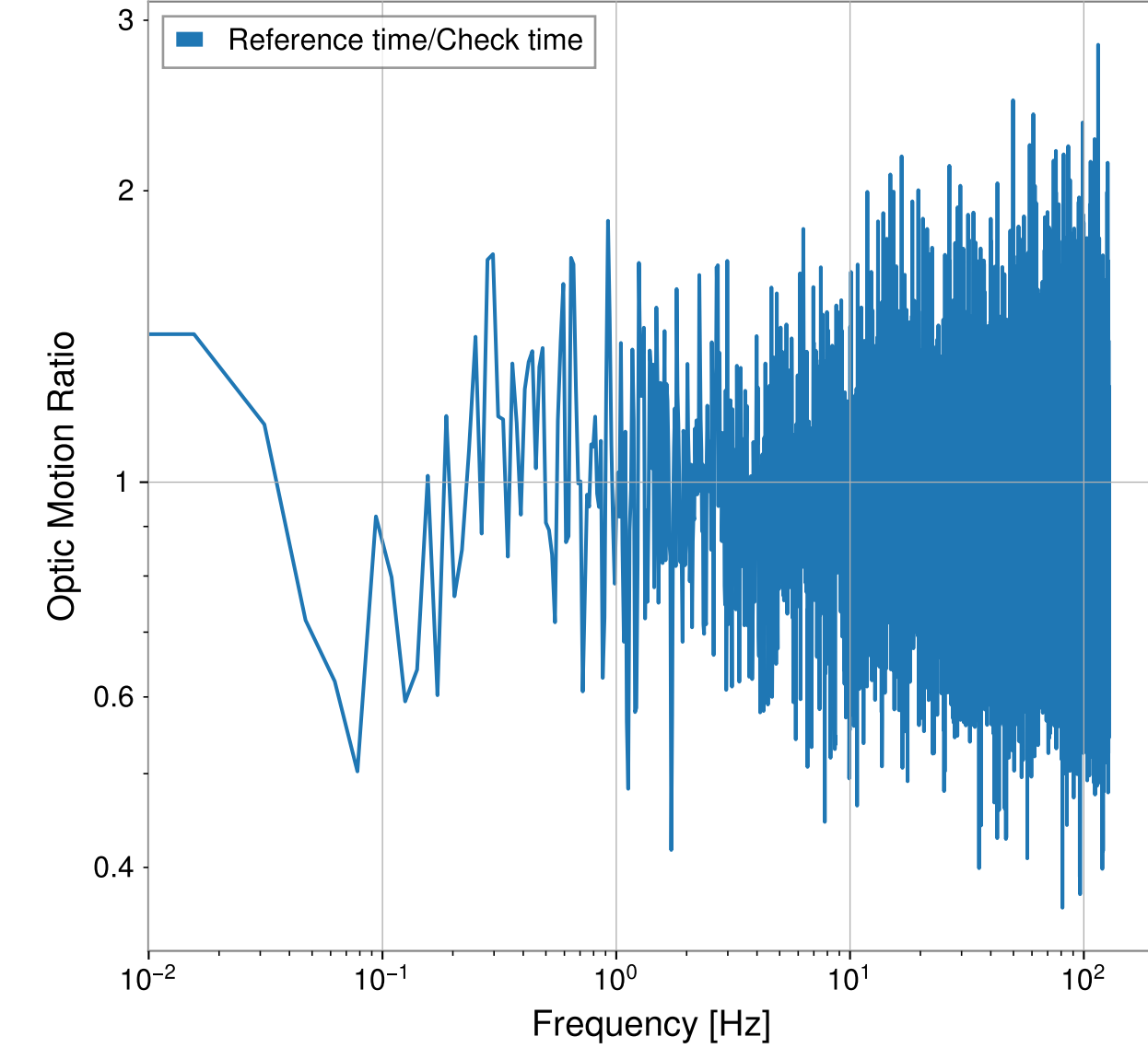
H1:SUS-TMSX_M1_DAMP_V_IN1_DQ
