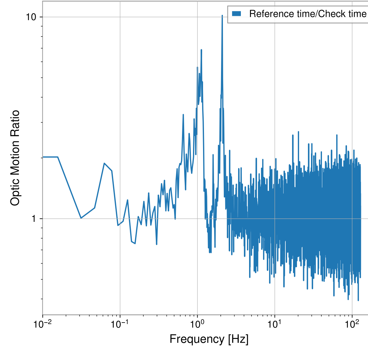
H1:SUS-MC3_M1_DAMP_Y_IN1_DQ
