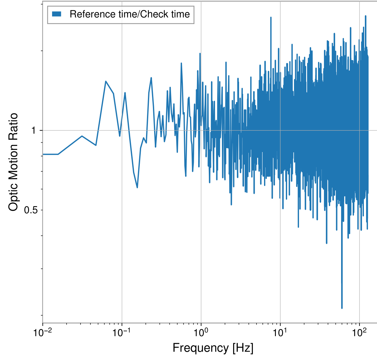
H1:SUS-MC3_M1_DAMP_P_IN1_DQ
