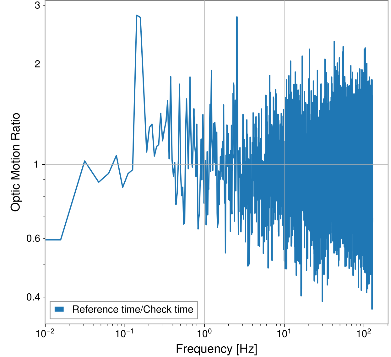
H1:SUS-TMSX_M1_DAMP_P_IN1_DQ
