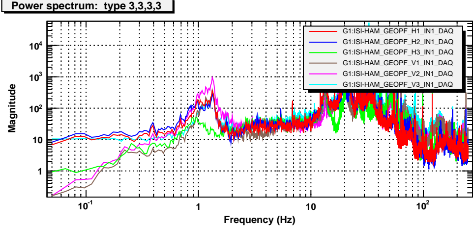
Power spectrum: type 3,3,3,3
