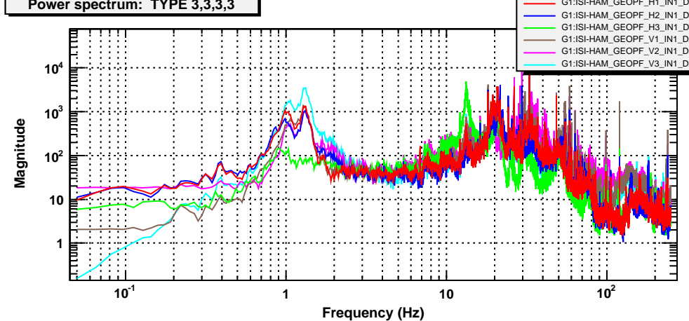
Power spectrum: TYPE 3,3,3
